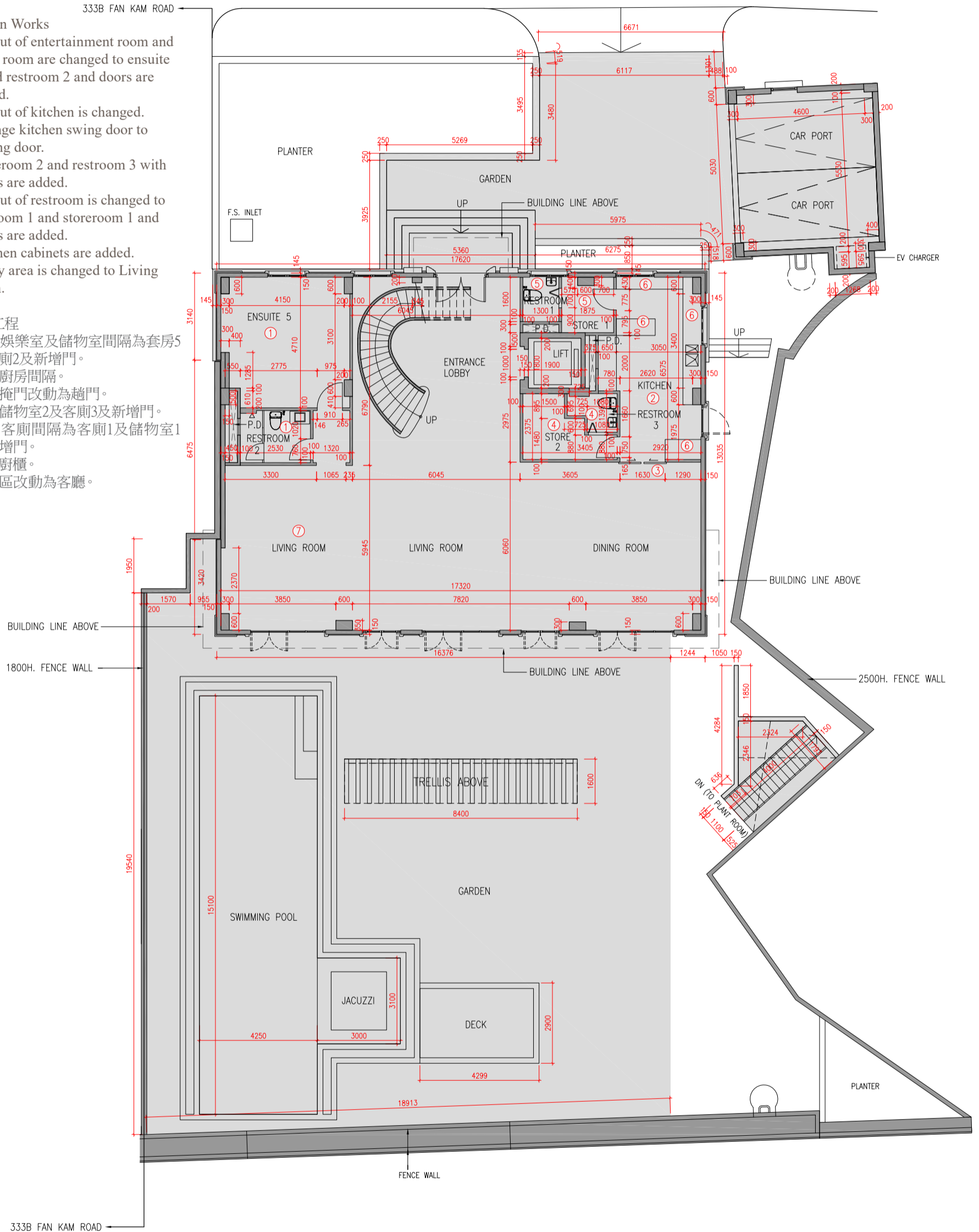
G/F AS-IS FLOOR PLAN 地下現狀平面圖
