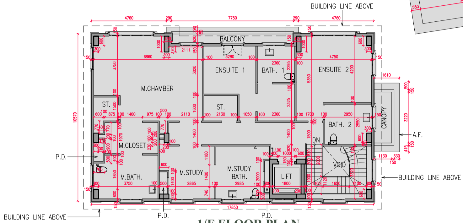
1/F FLOOR PLAN 1樓樓面平面圖
