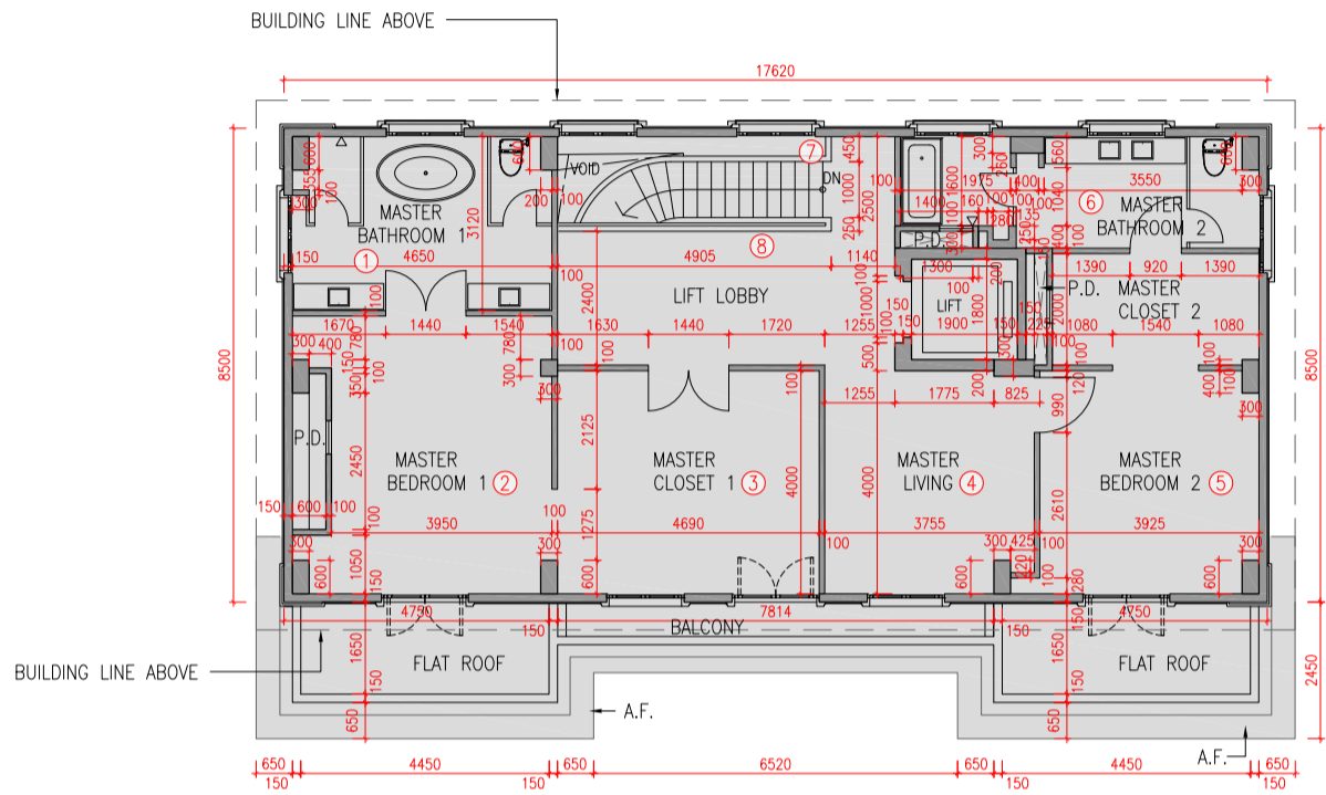
2/F AS-IS FLOOR PLAN 2樓現狀平面圖
